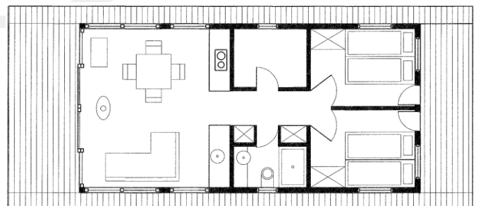
Grundriss Basisversion Vagabund 38
